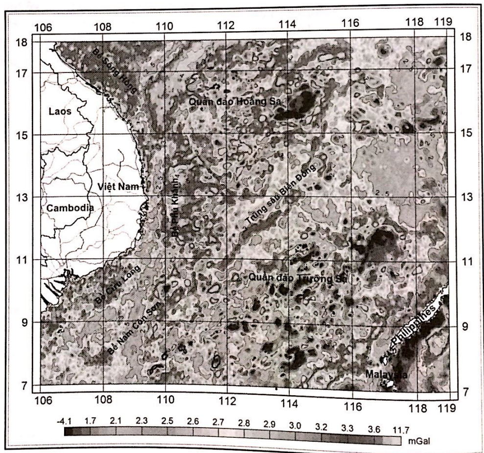
Hình 5. Sai lệch giữa dị thường trọng lực trước và sau khi áp dụng phương pháp bình phương tối thiểu collocation
