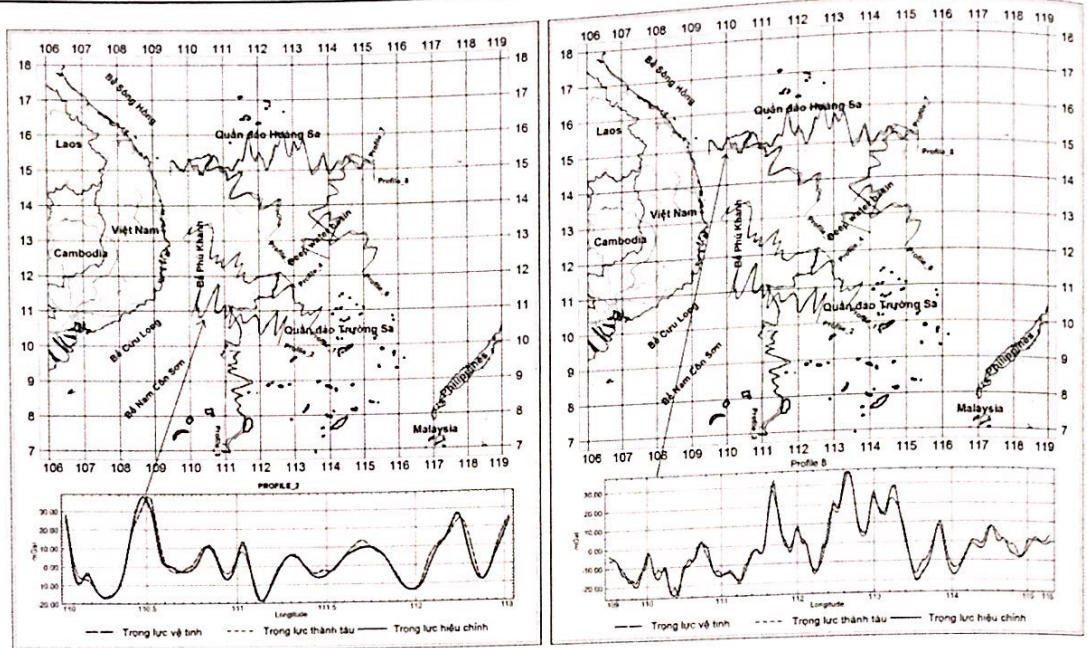
Hình 4. Các tuyến minh họa về hiệu chỉnh dị thường trọng lực vệ tinh dựa trên dị thường trọng lực thành tàu (tuyến 2, tuyến 8)
