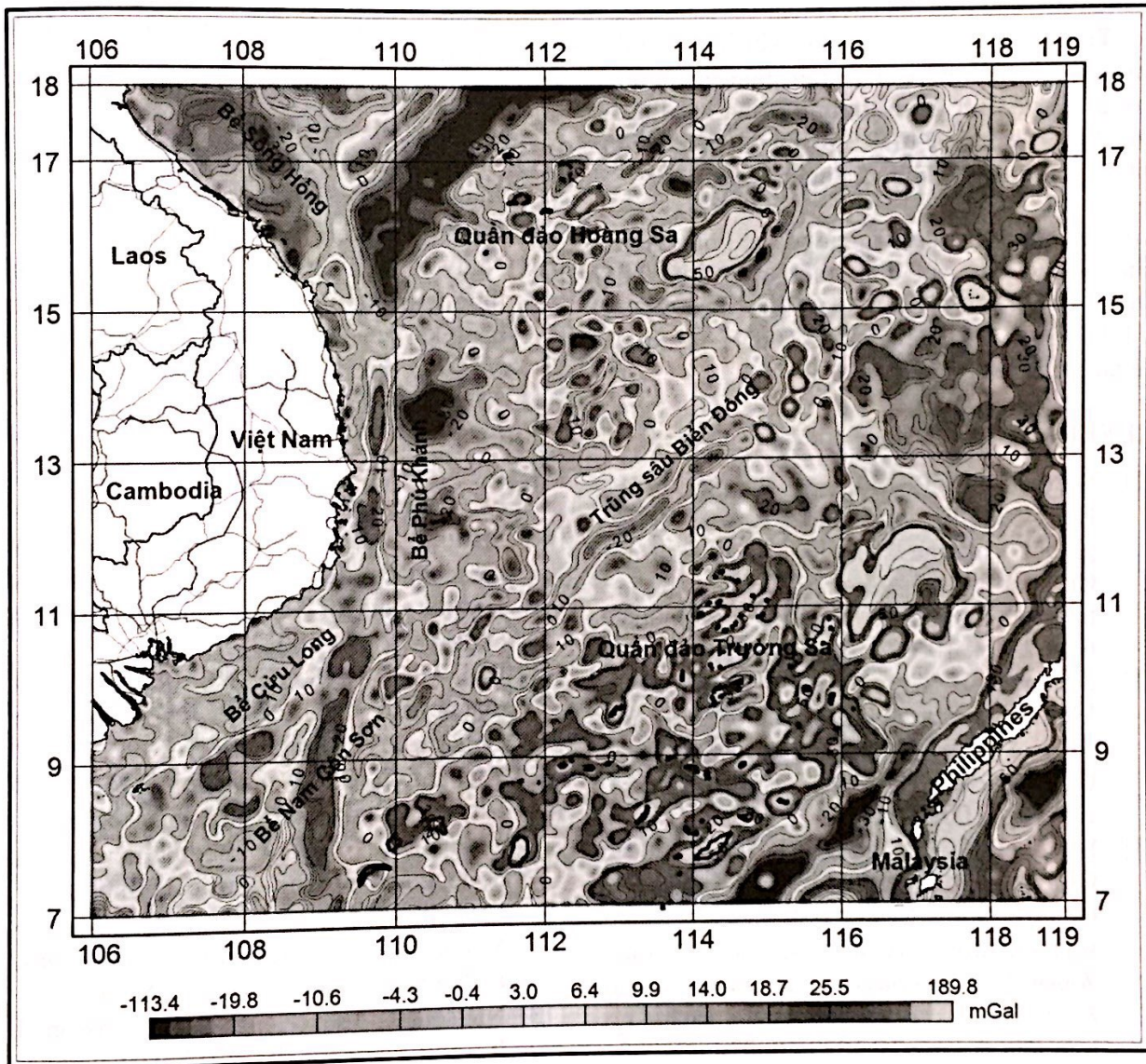
Hình 6. Dị thường trọng lực vệ tinh (Free_Air) đã được hiệu chỉnh
