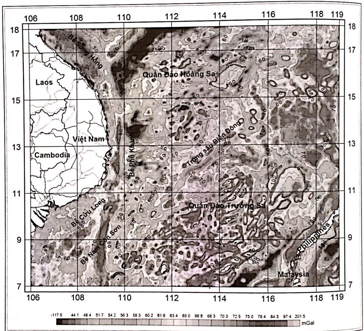
Hình 1. Dị thường trọng lực vệ tinh (Free-Air) [1]
