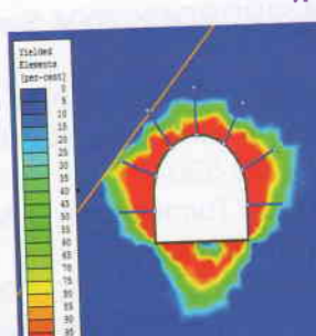
a) sử dụng mạng neo 09 cái
