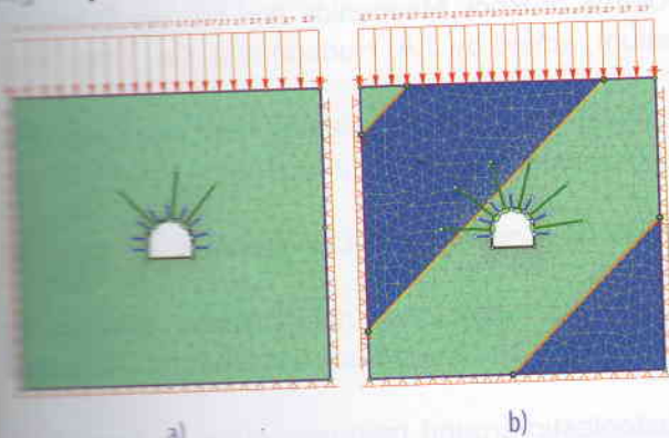
H.5. Sơ đồ mô hình số cho hai trường hợp phân tích: a) Trường hợp 1: đất đá đồng nhất sử dụng neo 02 mức: a) 09 neo ngắn và 03 neo cáp dài; b) Trường hợp 2: đất đá phân lớp sử dụng neo ngắn và 06 neo cáp dài
