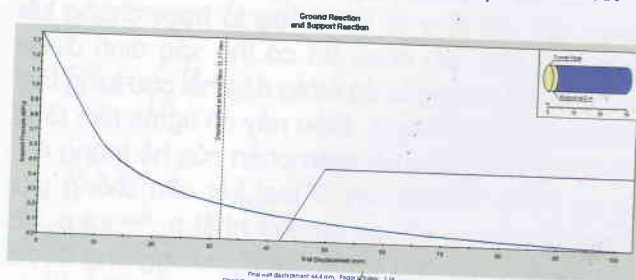
H.4. Ví dụ mô hình phân tích theo hệ số SF từ phần mềm Rocsupport 3.0
