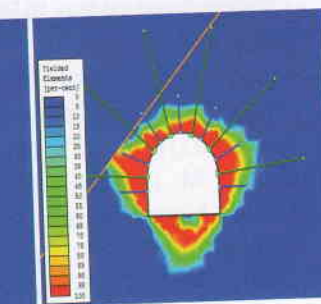
b) neo mạng kết hợp 06 neo cáp dài
