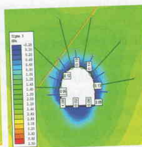
b) neo mạng với 06 neo cáp dài
