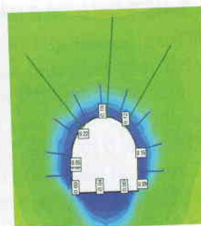
b) neo mạng với 03 neo cáp dài
