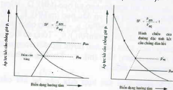
H.3. Định nghĩa thiết kế kết cấu chống theo hệ số an toàn SF
