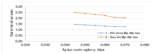
H.13. Biểu đồ quan hệ giữa áp lực nước ngầm p (MPa) và giá trị hệ số an toàn của khối nêm phía nóc số 8
