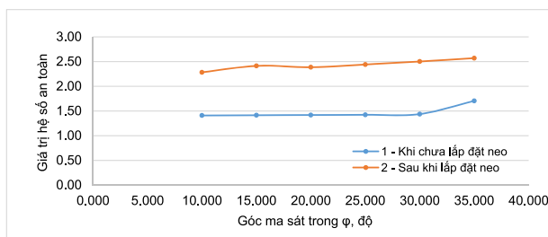
H.12. Biểu đồ quan hệ giữa góc ma sát phi (độ) và giá trị hệ số an toàn của khối nêi phía nóc số 8
