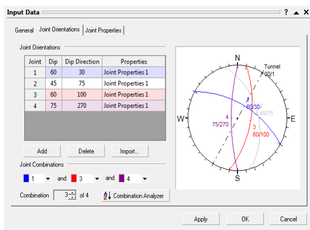
H.7. Vị trí tương đối trục đường hầm và các khe nứt
