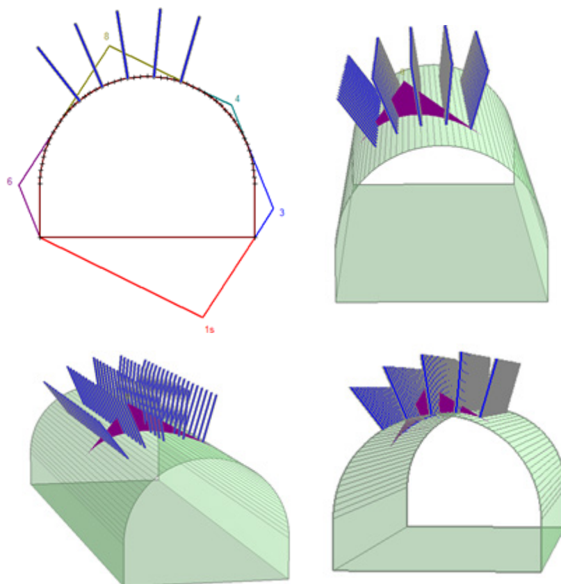
H10. Gia cố vì neo giữ ổn định khối nêi phía nóc số 8
