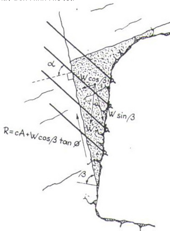
H.5. Gia cố khối nêm trượt
