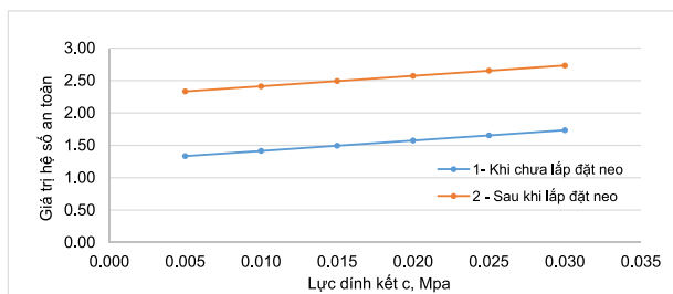
H.11. Biểu đồ quan hệ giữa lực đỉnh kết c (MPa) và Giá trị hệ số an toàn của khối nêi phía nóc số 8
