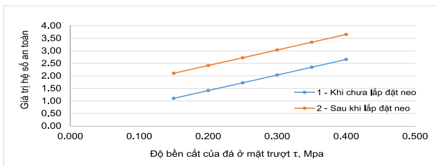
H.15. Biểu đồ quan hệ giữa độ bền cắt của đá ở mặt trượt \tau (MPa) và giá trị hệ số an toàn của khối nêm phía nóc số 8
