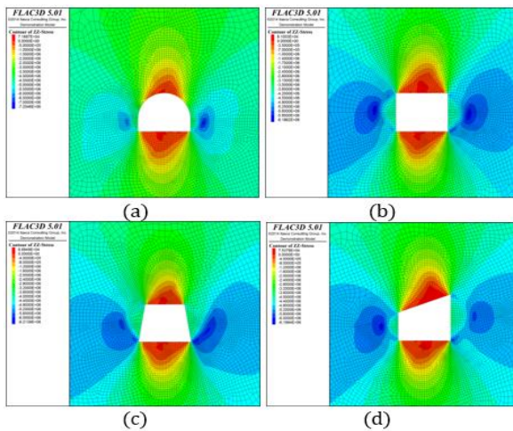
Hình 3. Phân bố ứng suất thẳng đứng khối đá xung quanh đường lò.
