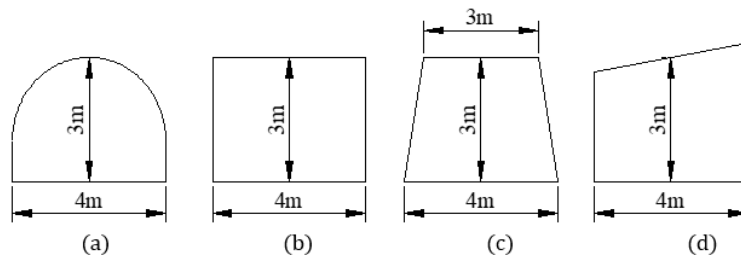
Hình 1. Bốn dạng mặt cắt ngang đường lò.
