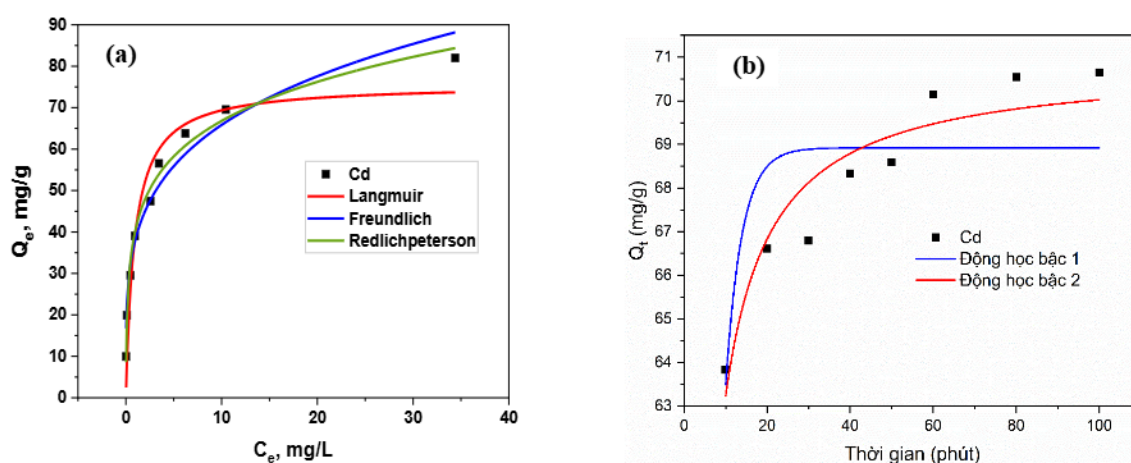
Hình 3: Đường đẳng nhiệt hấp phụ của Cd^{2+} theo mô hình Langmuir, Freundlich và Redlich–Peterson (a) và động học của quá trình hấp phụ Cd^{2+} lên HAP theo phương trình giả bậc 1 và giả bậc 2 (b)
