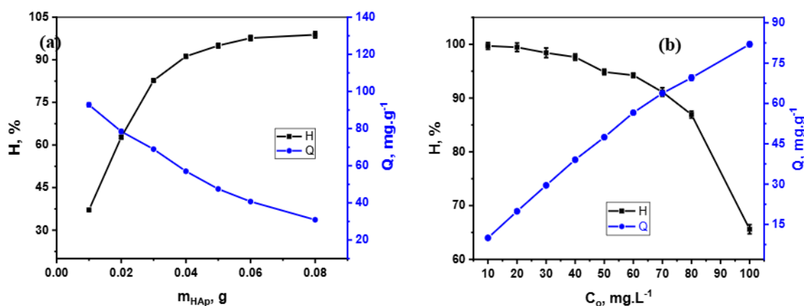
Hình 2: Ảnh hưởng của khối lượng bột HAP ( C = 50 mg/L, t = 60 phút; pH = 6,48 , T = 25 °C) (a) và nồng độ Cd^{2+} ban đầu ( m_{HAP} = 0,05 g, t_{tiếp xúc} = 60 phút; pH = 6,48 , T = 25 °C) (b) đến khả năng hấp phụ của HAP
