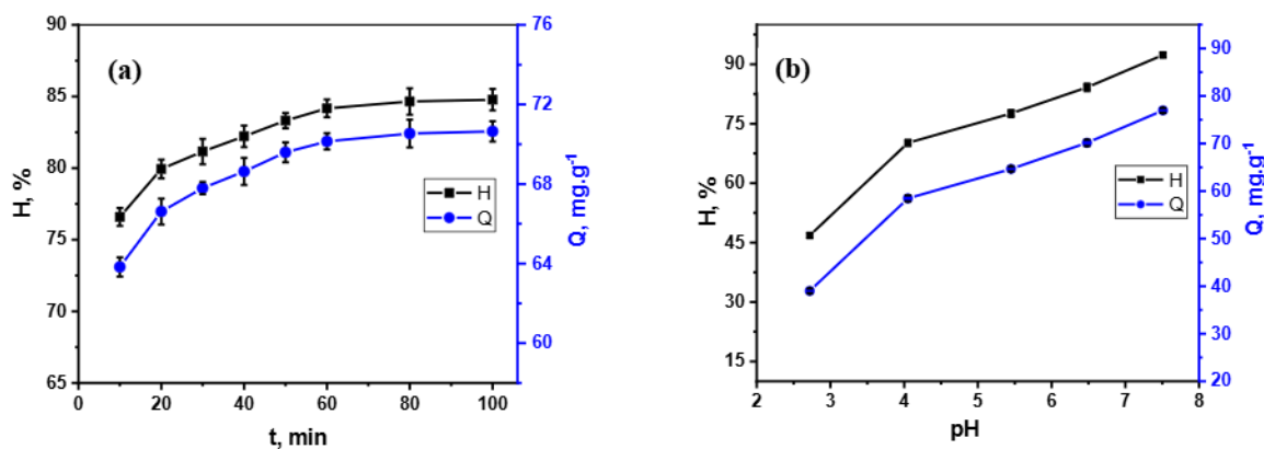
Hình 1: Ảnh hưởng của thời gian tiếp xúc ( C_{Cd^{2+}} = 50 mg/L, m = 0,03 g, pH = 6,48, T = 25^\circ C ) (a) và pH ( C_{Cd^{2+}} = 50 mg/L, m_{HAP} = 0,03 g, t = 60 phút, T = 25^\circ C ) (b) đến khả năng hấp phụ Cd^{2+}
