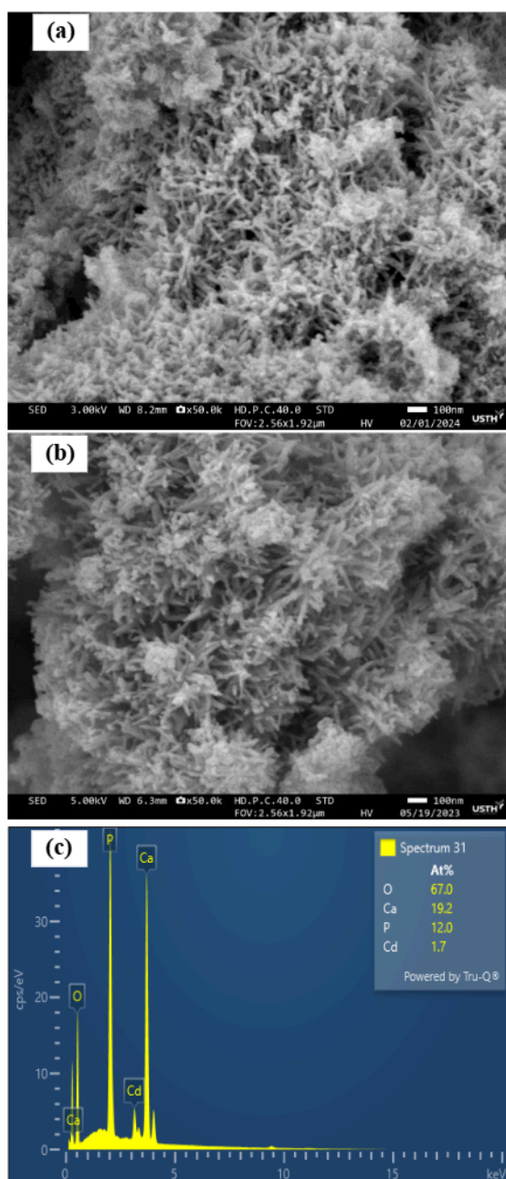
Hình 4: Hình ảnh SEM của vật liệu HAp ban đầu (a), HAp sau hấp phụ Cd 2+ (b) và EDX của HAp sau hấp phụ Cd 2+ (c)
