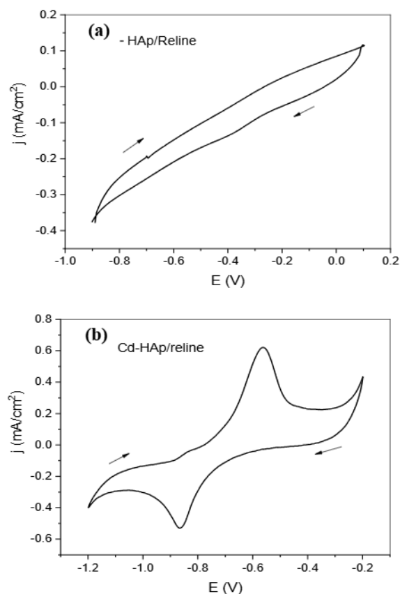
Hình 5: Đường CV của HAp (a) và Cd-HAp (b) trong Reline
