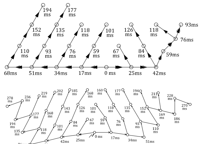
H.6. Sơ đồ vi sai sử dụng tại hai vụ nổ HS1 (trái) và HS2 (phải)
